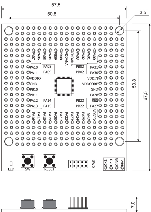
Рис. 1. Габаритные размеры
