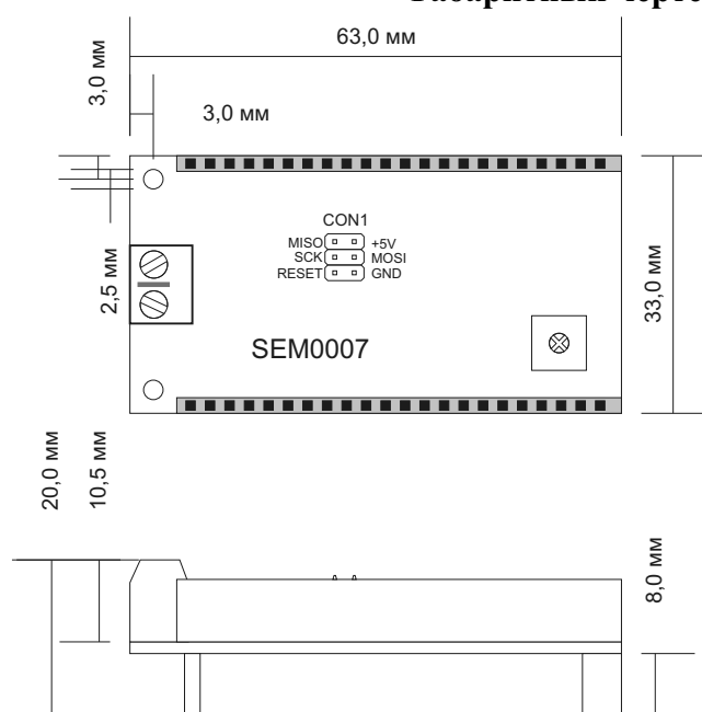
Габаритный чертеж
