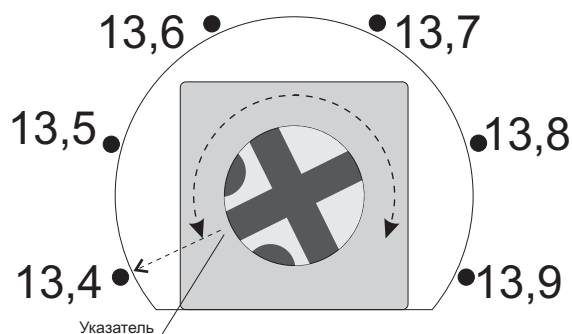
Рис. 3. Регулировка напряжения окончания заряда
