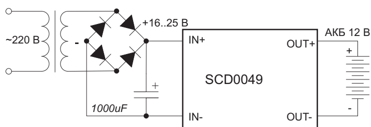
Рис. 1. Схема включения
