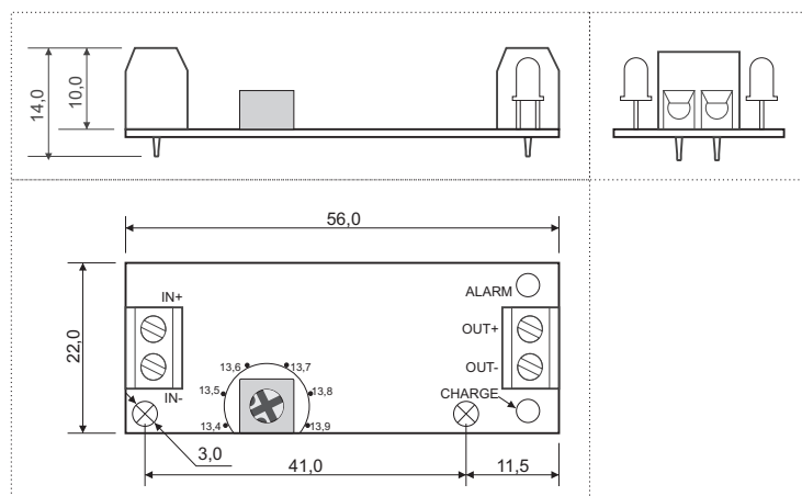
Рис. 2. Габаритные размеры
