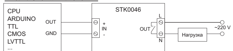
Рис. 1. Схема включения
