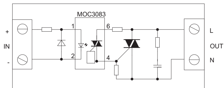
Рис. 2. Схема модуля
