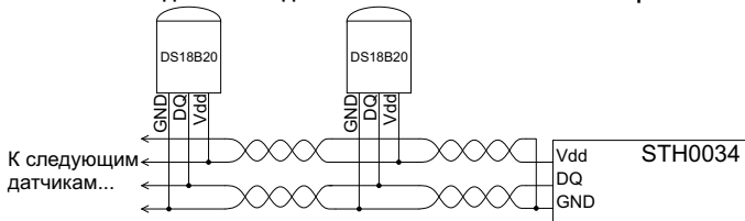
Рис. 6. Схема подключения датчиков с использованием 2-х парной витой пары.
