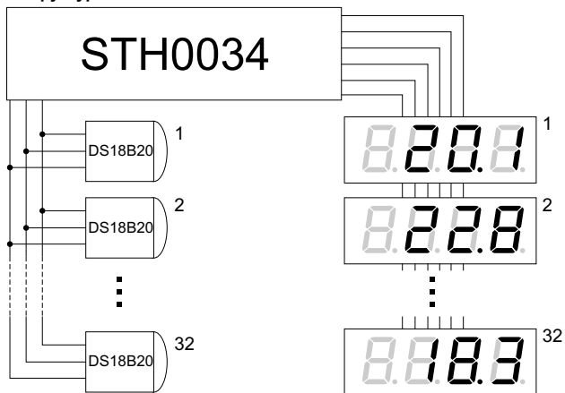
Рис. 3. Структурная схема
