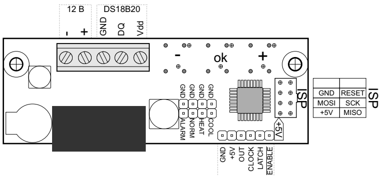
Рис. 1. Распиновка контактов
