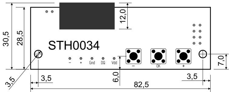
Рис. 2. Габаритный чертеж
