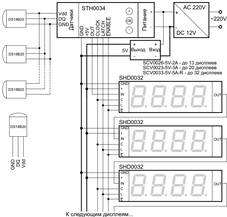
Рис. 6. Схема подключения датчиков с использованием 2-х парной витой пары.
