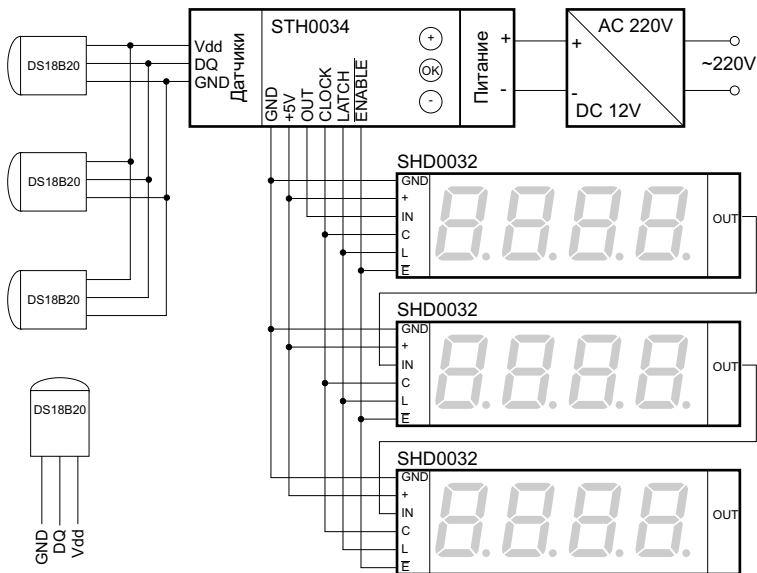
Рис. 4. Схема включения для трех дисплеев и менее.
