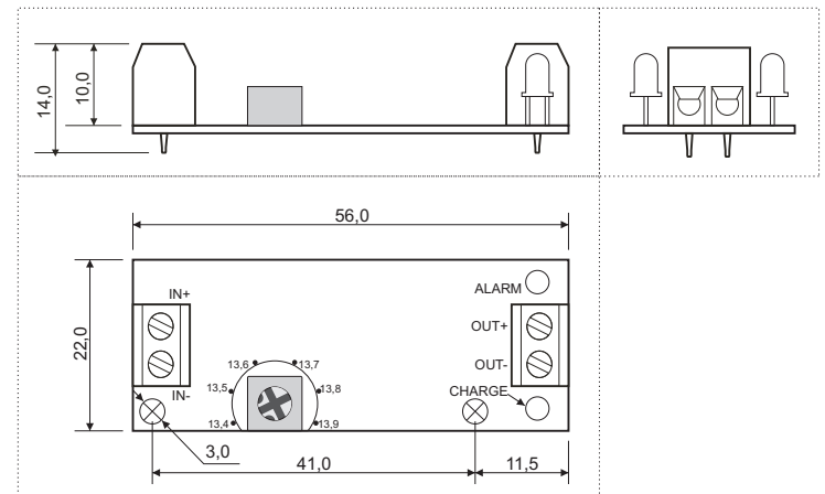
Рис. 2. Габаритные размеры
