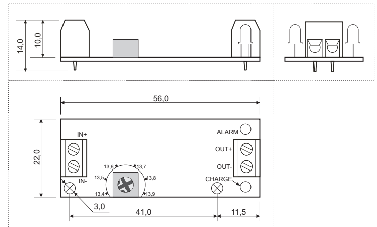
Рис. 2. Габаритные размеры
