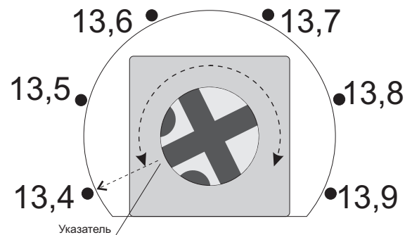
Рис. 3. Регулировка напряжения окончания заряда
