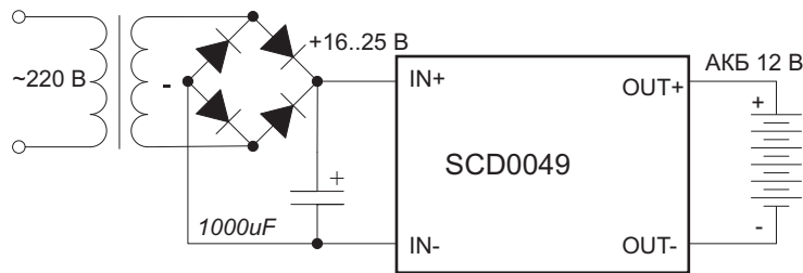
Рис. 1. Схема включения
